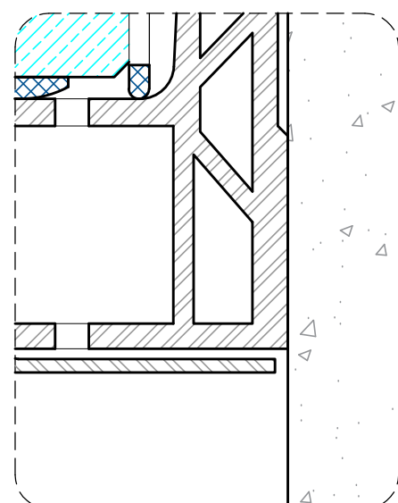
Detail A. Drainage Scale 1:4
